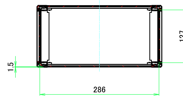
A-A ( 1 : 5.5 )
