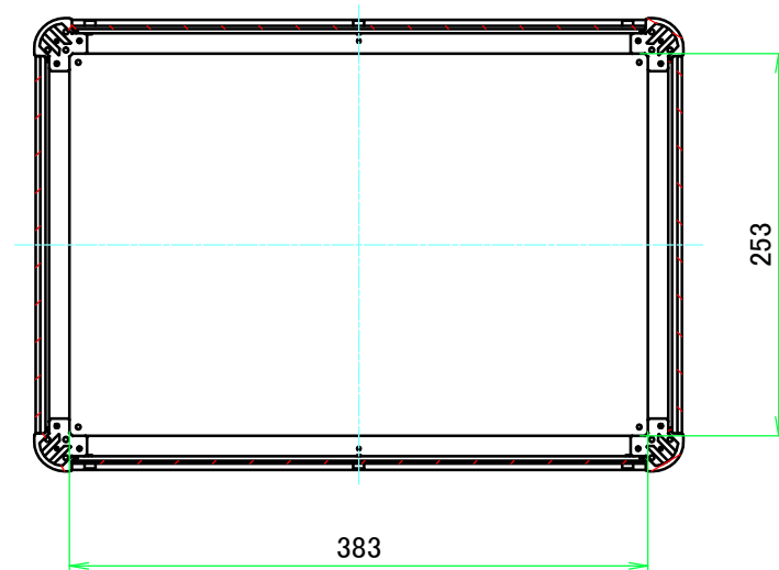
B-B ( 1 : 5.5 )
