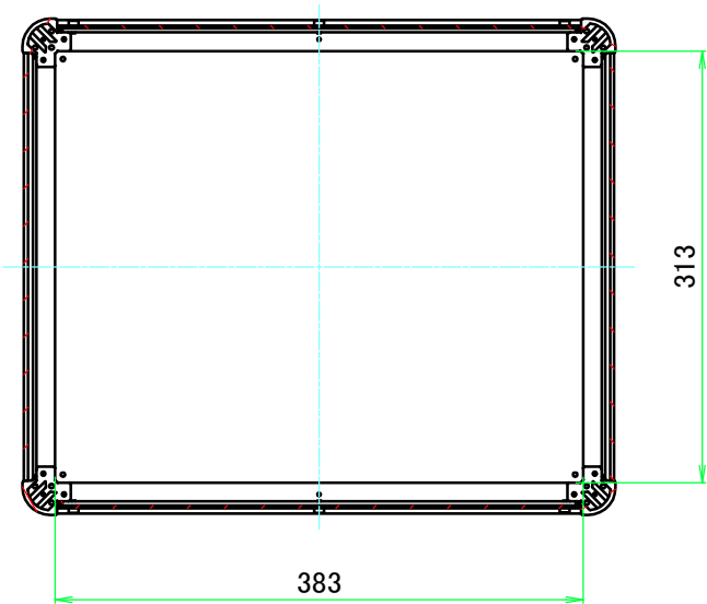
B-B ( 1 : 6 )
