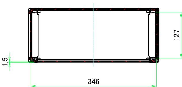
A-A ( 1 : 6 )
