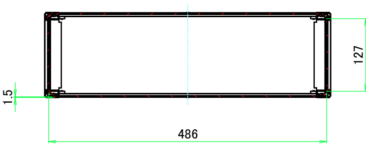
A-A ( 1 : 6.5 )
