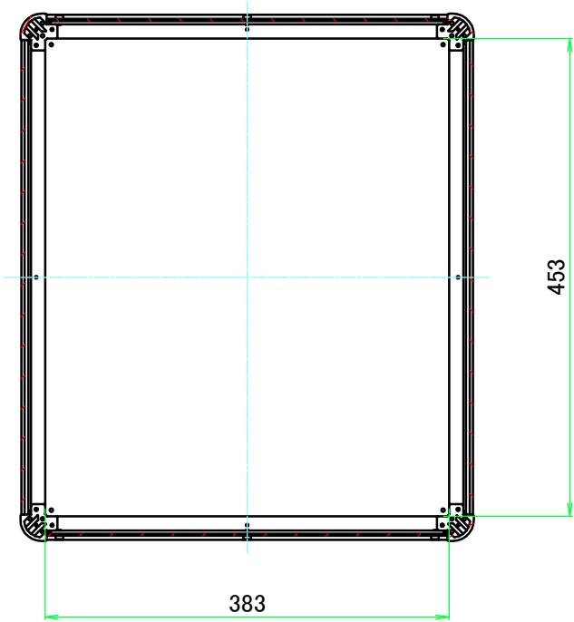
B-B ( 1 : 6.5 )
