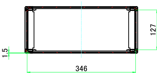
A-A ( 1 : 7 )
