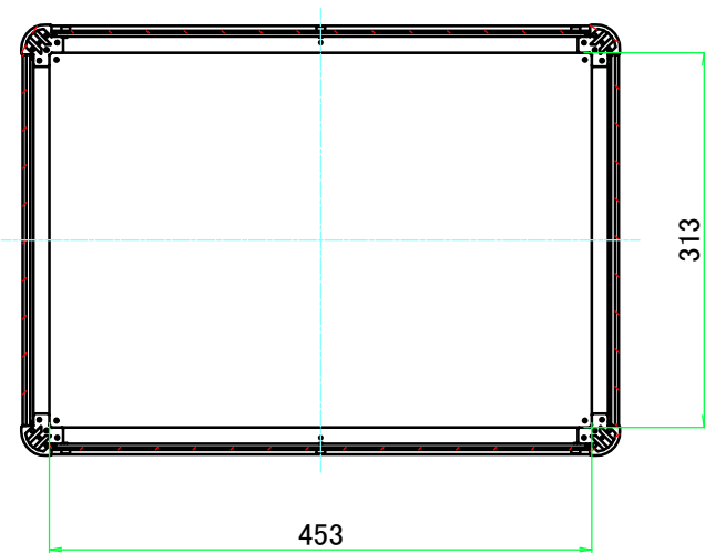
B-B ( 1 : 7 )
