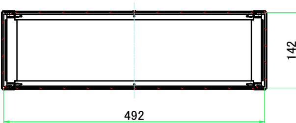
C-C ( 1 : 7 )
