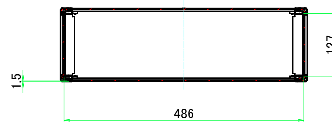
A-A ( 1 : 7.5 )
