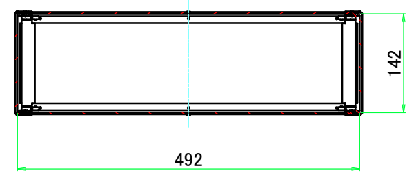
C-C ( 1 : 7.5 )
