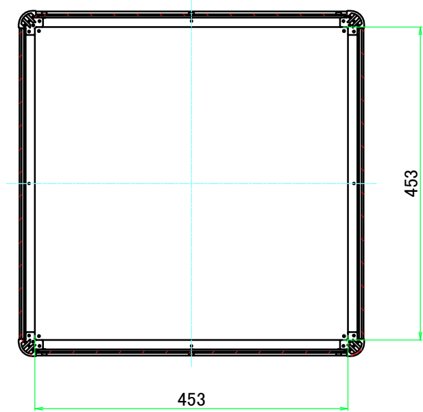
B-B ( 1 : 7.5 )
