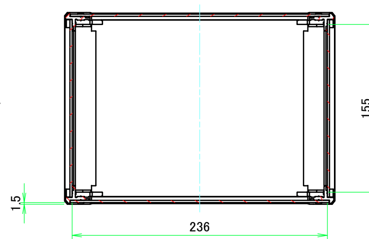
A-A ( 1 :3.5 )
