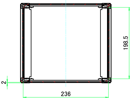
A-A ( 1 : 5 )
