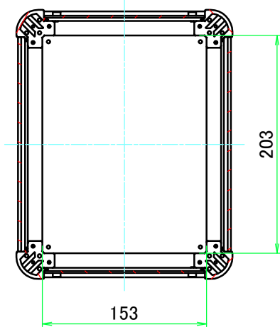
B-B ( 1 : 5 )
