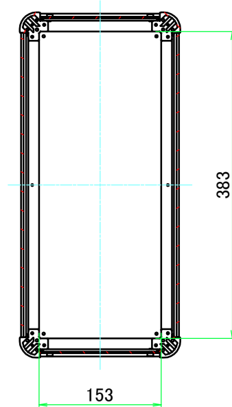
B-B ( 1 : 6.5 )
