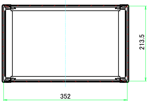
C-C ( 1 : 5.5 )
