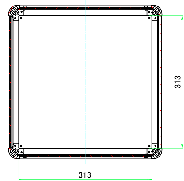
B-B ( 1 : 5.5 )
