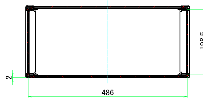
A-A (1:7)
