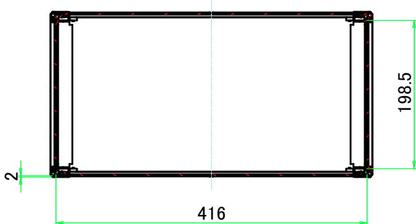
A-A ( 1 : 7 )
