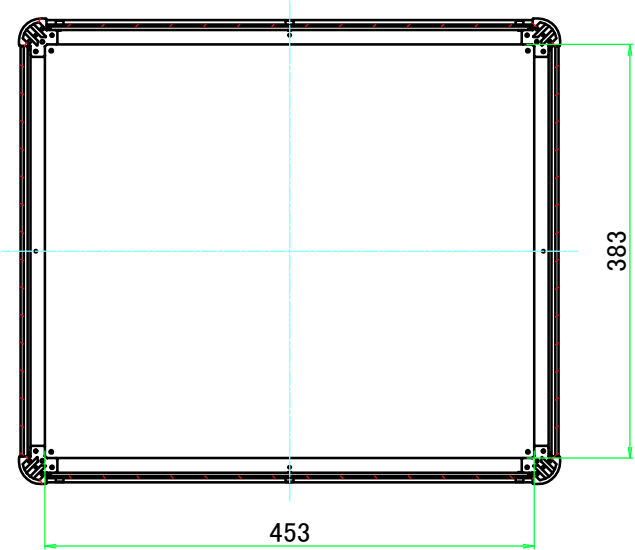
B-B ( 1 : 7 )
