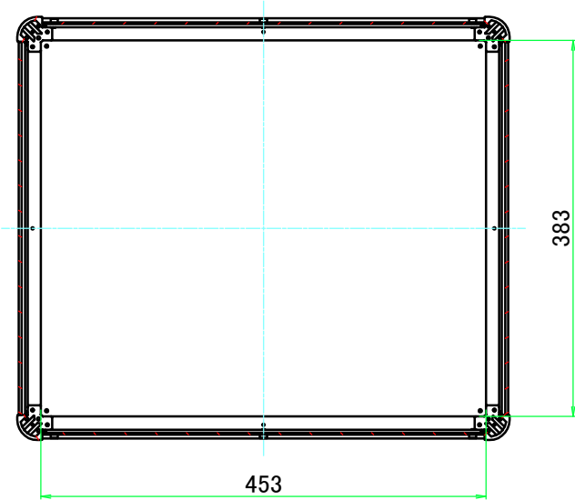
B-B ( 1 : 7 )
