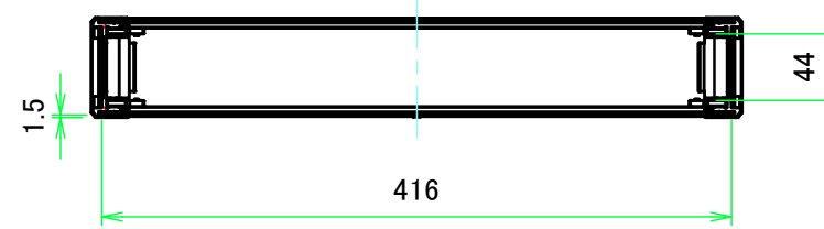
A-A ( 1:5.5 )
