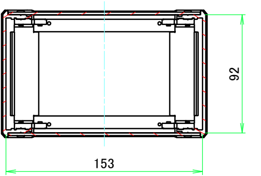
C-C ( 1 : 3 )
