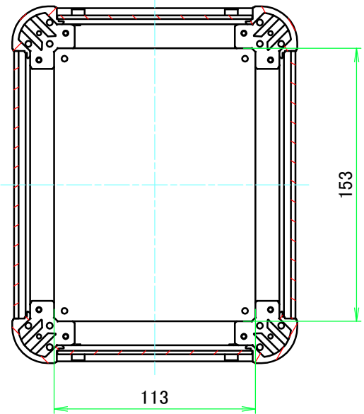
B-B ( 1 : 3 )
