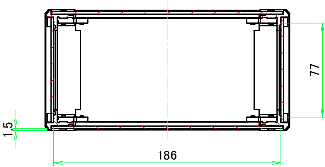
A-A ( 1 : 3 )
