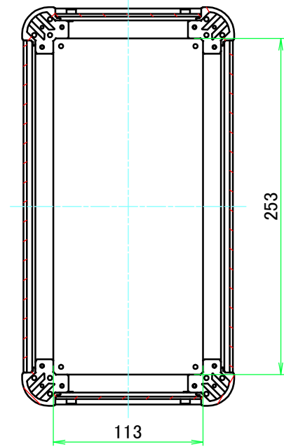
B-B ( 1 : 4 )
