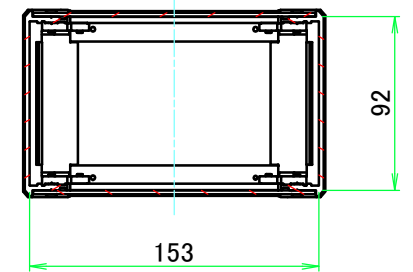
C-C ( 1 : 4 )
