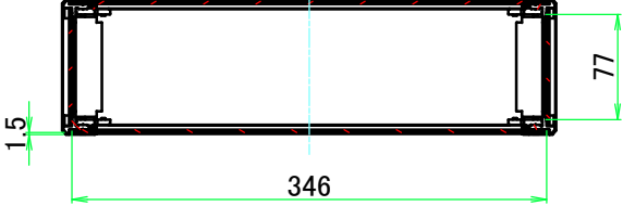
A-A ( 1 : 6 )
