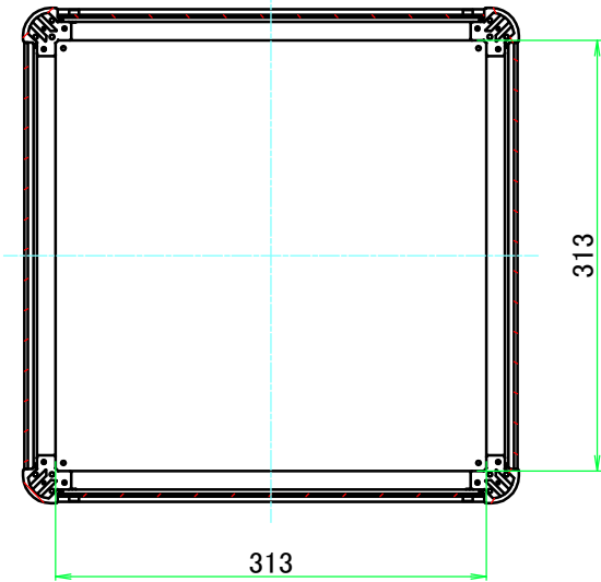
B-B ( 1 : 6 )
