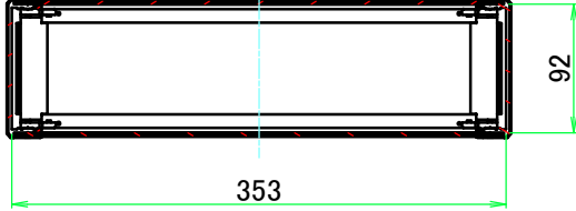
C-C ( 1 : 6 )
