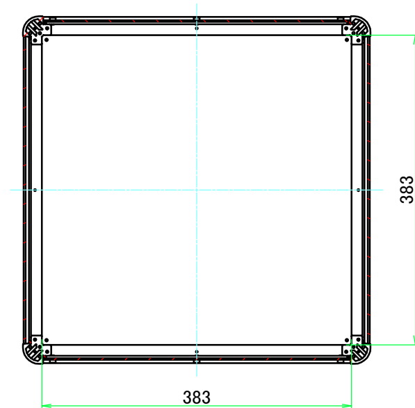
B-B ( 1 : 6.5 )
