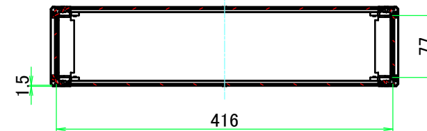
A-A ( 1 : 6.5 )
