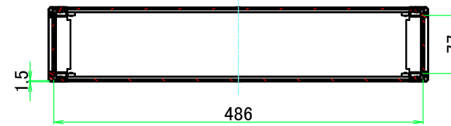
A-A (1:7)
