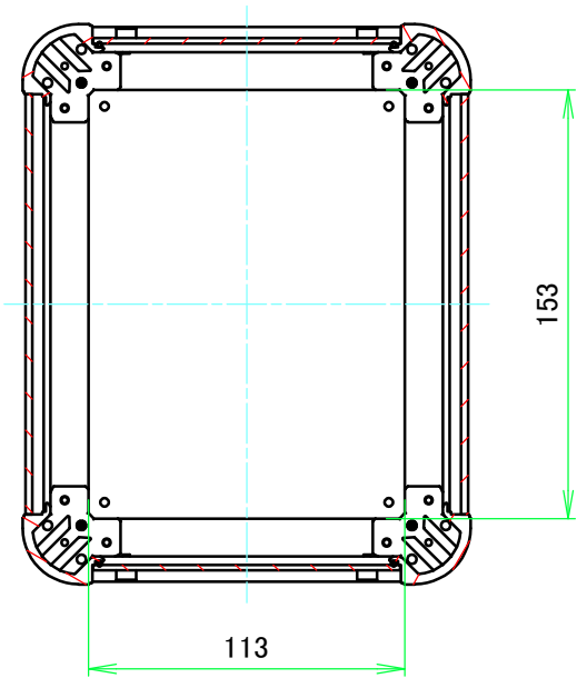
B-B ( 1 : 3 )
