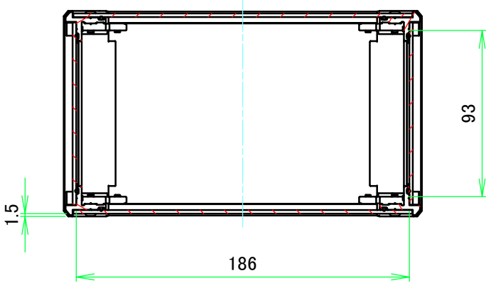
A-A ( 1 : 3 )
