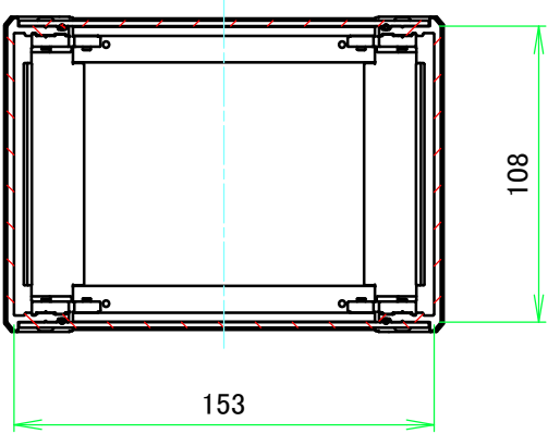
C-C ( 1 : 3 )
