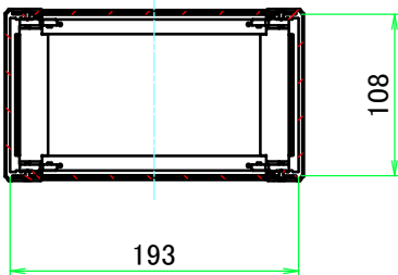
C-C ( 1 : 5.5 )
