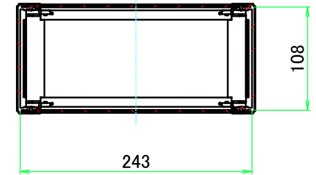
C-C ( 1 : 5.5 )
