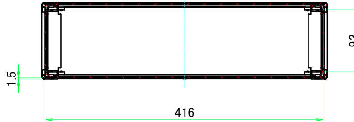
A-A ( 1 : 5.5 )
