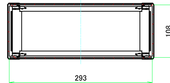
C-C ( 1 : 4.5 )
