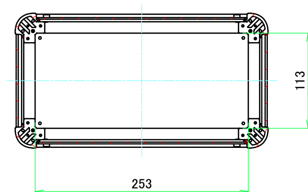
B-B ( 1 : 4.5 )
