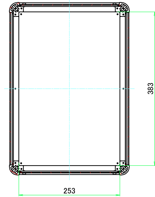
B-B ( 1 : 5.5 )
