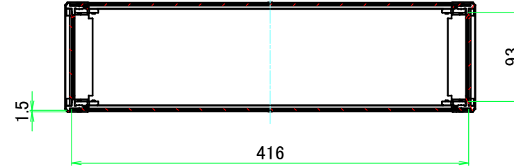
A-A ( 1 : 5.5 )
