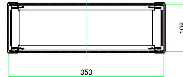
C-C ( 1 : 5 )
