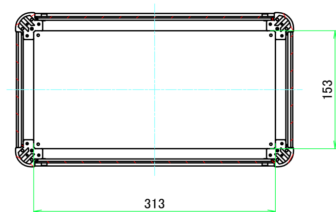
B-B ( 1 : 5 )
