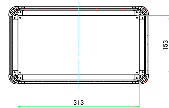
B-B ( 1 : 5 )
