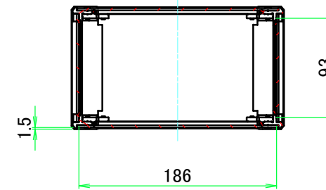
A-A ( 1 : 5 )
