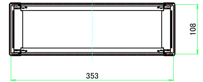
C-C ( 1 : 5 )
