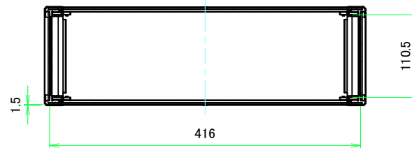
A-A (1:5)
