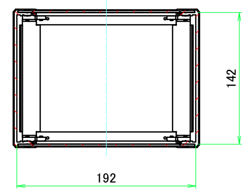
C-C ( 1 : 4 )
