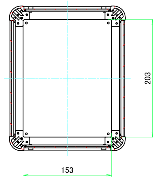
B-B ( 1 : 4 )
