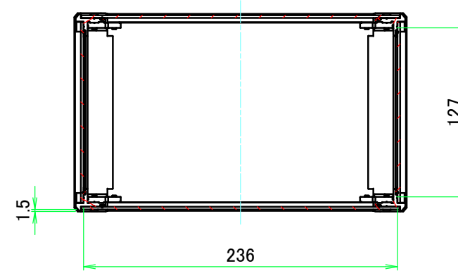
A-A ( 1 : 4 )
