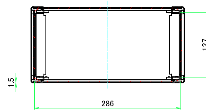
A-A ( 1 : 4.5 )
