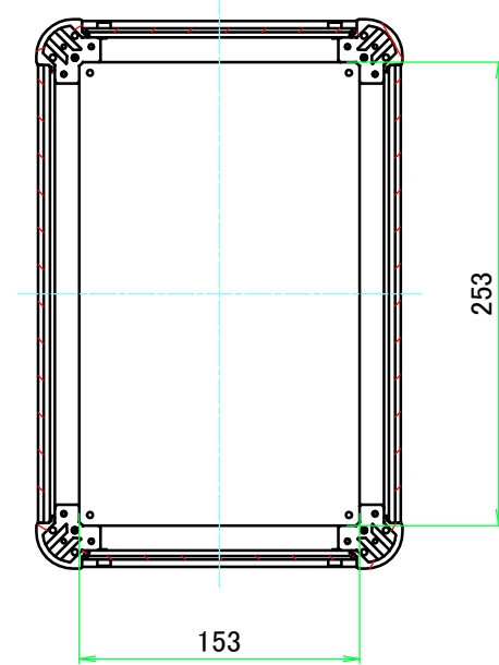
B-B ( 1 : 4.5 )
