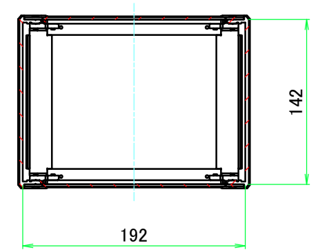
C-C ( 1 : 4.5 )
