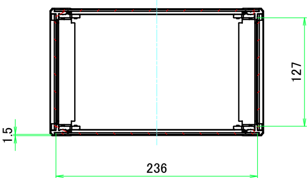
A-A ( 1 : 4.5 )
