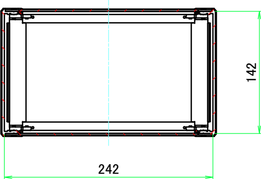
C-C ( 1 : 4.5 )
