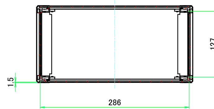
A-A ( 1 : 4.5 )
