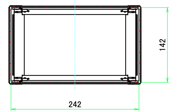
C-C ( 1 : 4.5 )
