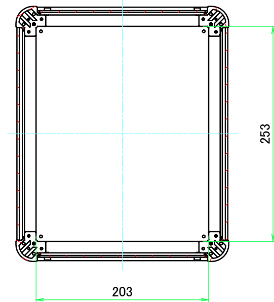
B-B ( 1 : 4.5 )
