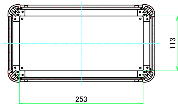
B-B ( 1 : 4.5 )
