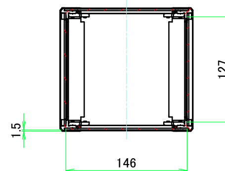
A-A ( 1 : 4.5 )
