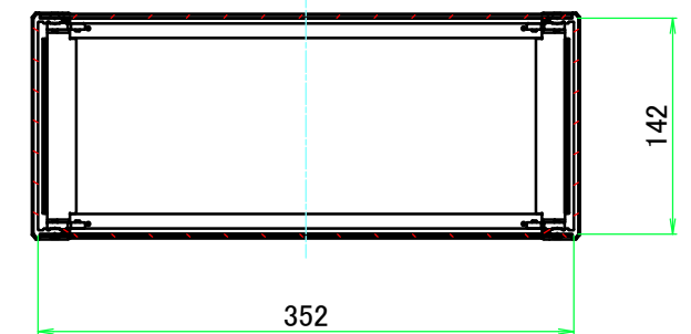
C-C ( 1 : 5.5 )
