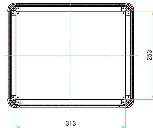
B-B ( 1 : 5.5 )
