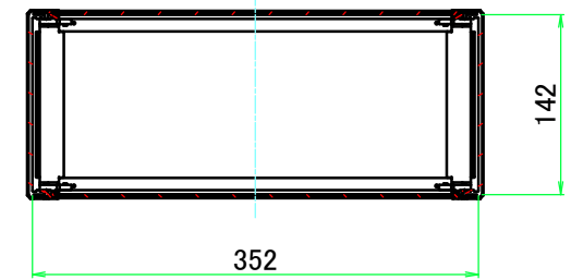
C-C ( 1 : 6.5 )
