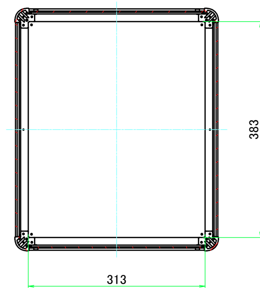
B-B ( 1 : 6.5 )
