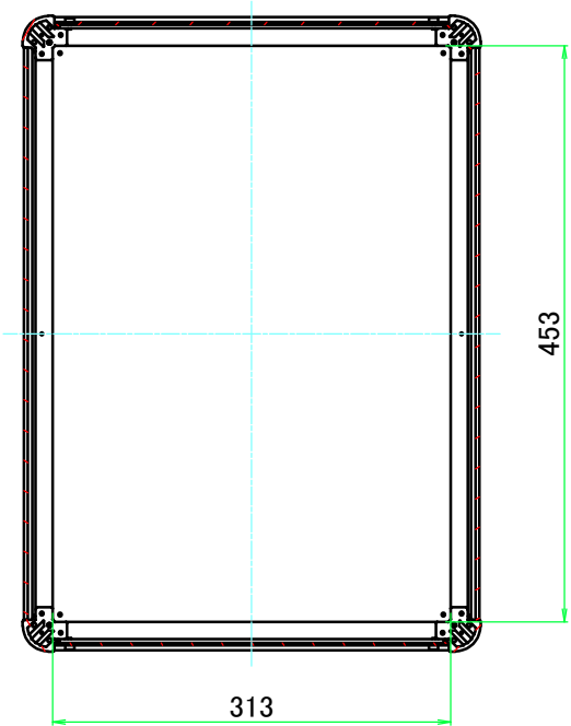
B-B ( 1 : 6.5 )
