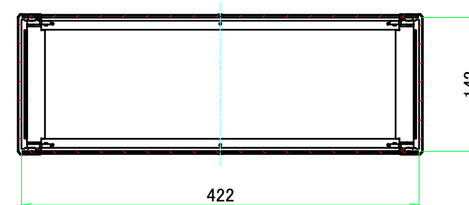
C-C ( 1 : 5.5 )
