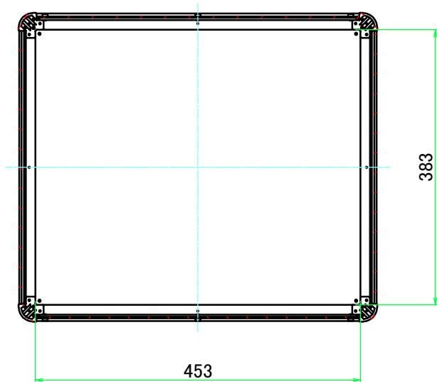
B-B ( 1 : 7.5 )
