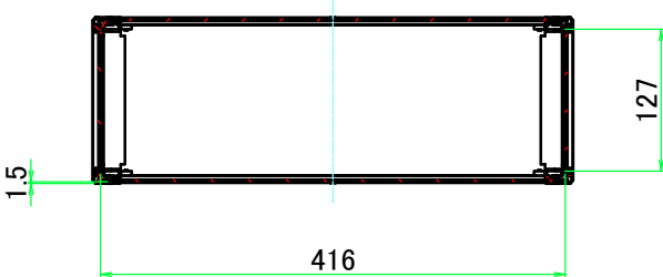
A-A ( 1 : 7.5 )
