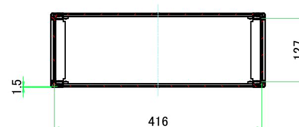
A-A ( 1 : 7.5 )
