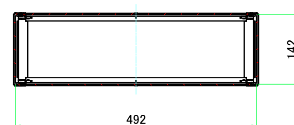
C-C ( 1 : 7.5 )
