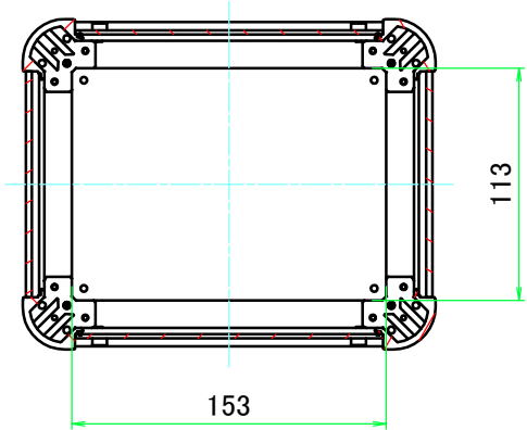
B-B ( 1 : 4 )
