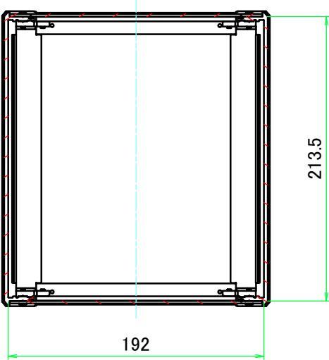
C-C ( 1 : 4 )
