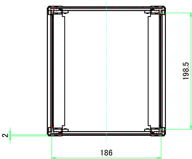
A-A ( 1 : 4 )
