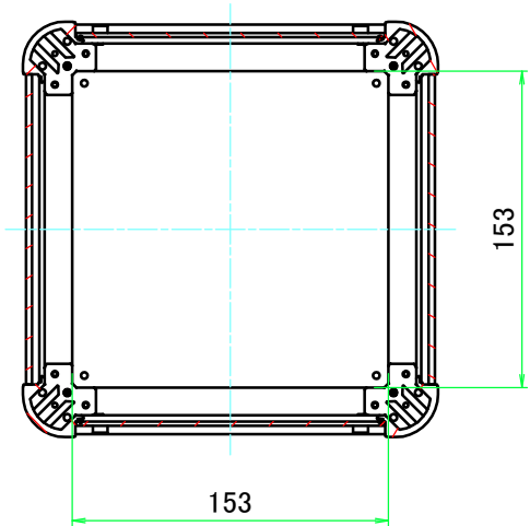
B-B ( 1 : 4 )
