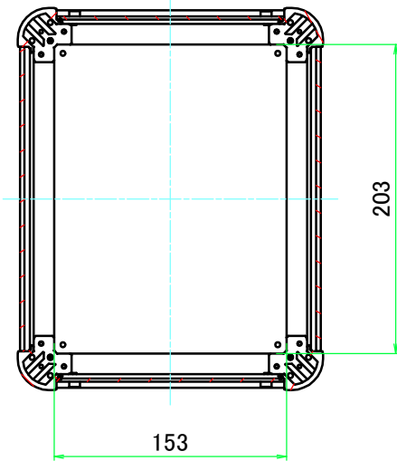
B-B ( 1 : 4.5 )
