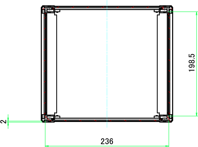
A-A ( 1 : 4.5 )
