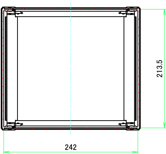
C-C ( 1 : 4 )
