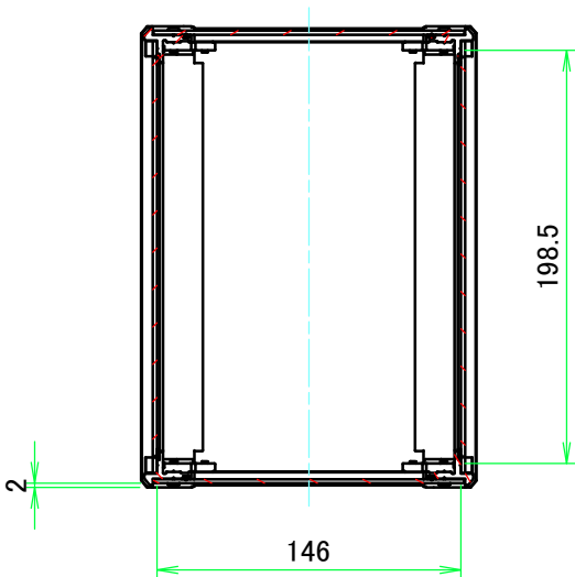
A-A ( 1 : 4 )
