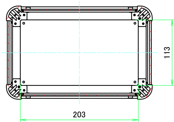
B-B ( 1 : 4 )
