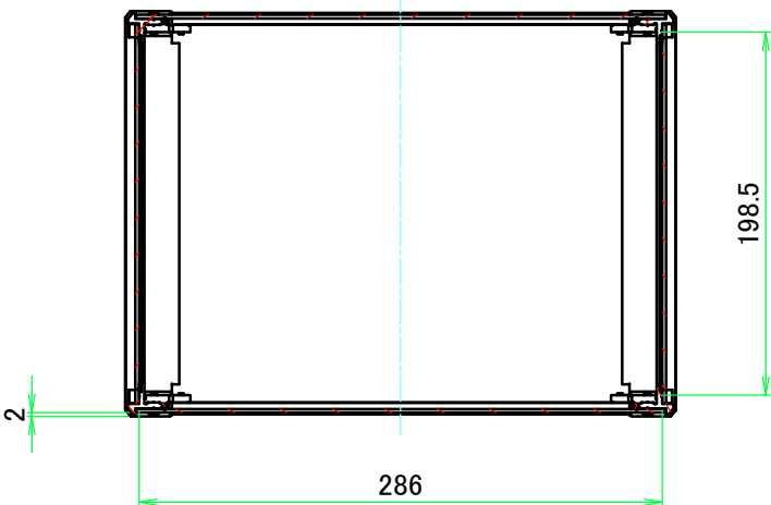
A-A ( 1 : 4.5 )
