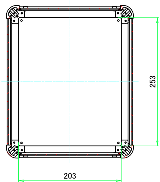
B-B ( 1 : 4.5 )
