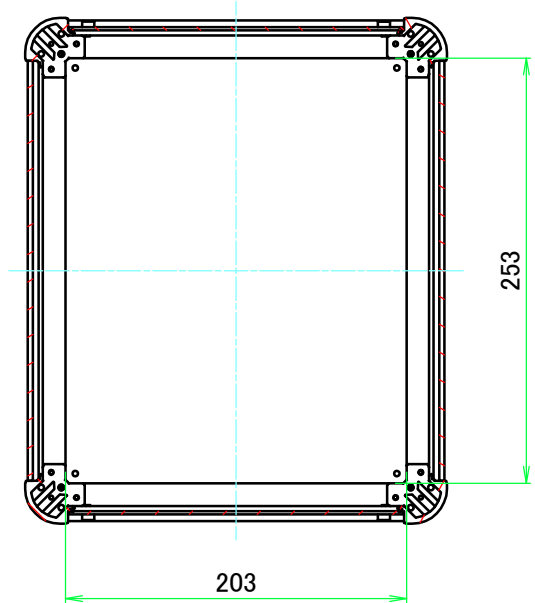
B-B ( 1 : 4.5 )
