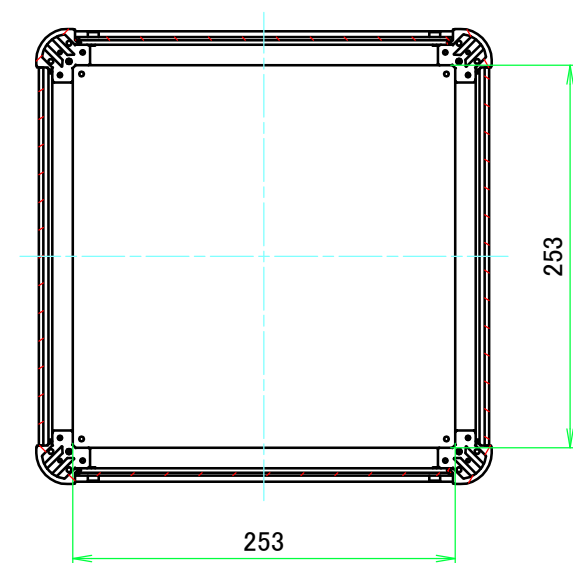
B-B ( 1 : 5 )
