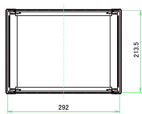
C-C ( 1 : 5 )
