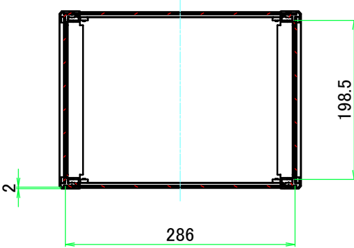
A-A ( 1 : 6.5 )
