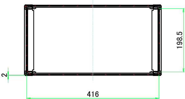
A-A ( 1 : 7 )
