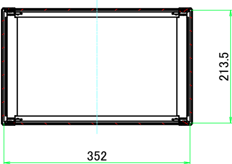
C-C ( 1 : 7 )
