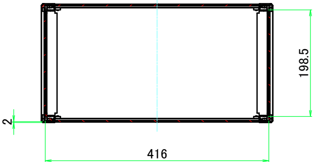
A-A ( 1 : 7 )
