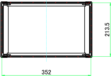
C-C ( 1 : 7 )
