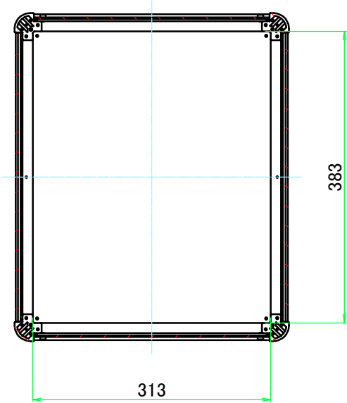
B-B ( 1 : 7 )
