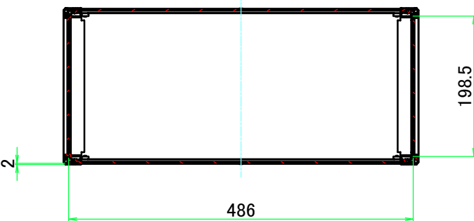
A-A ( 1 : 7.5 )
