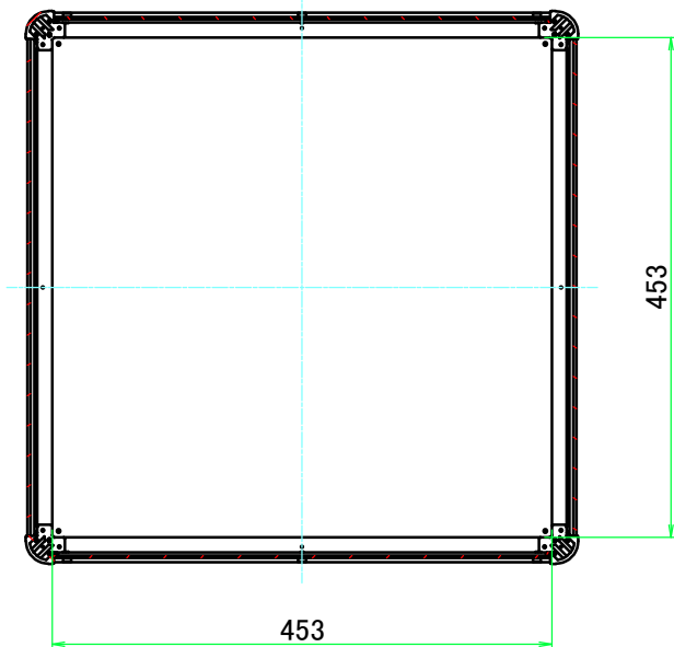
B-B ( 1 : 7.5 )
