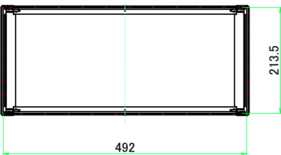
C-C ( 1 : 7.5 )
