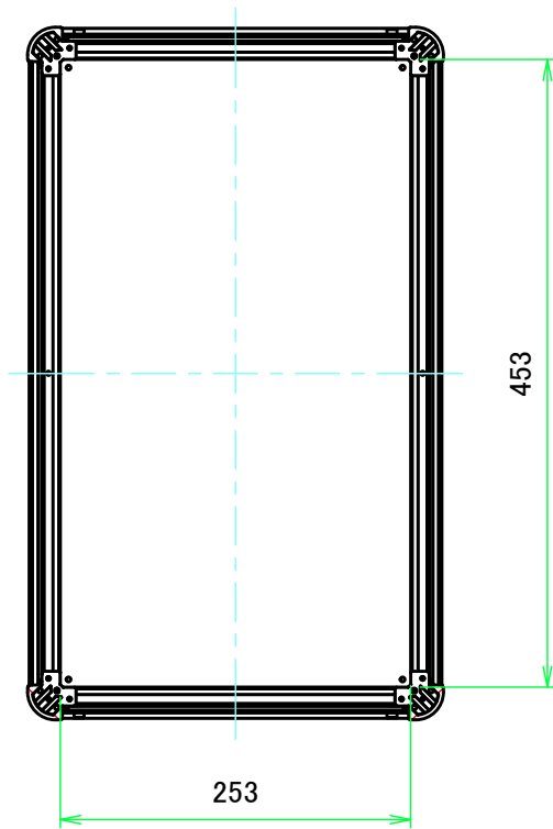
B-B ( 1:6 )
