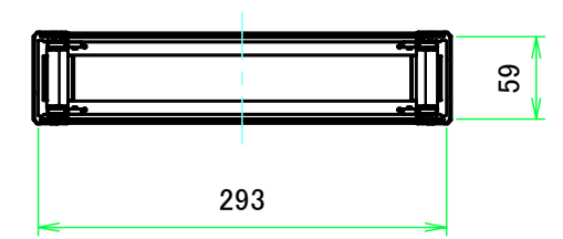
C-C ( 1:6 )
